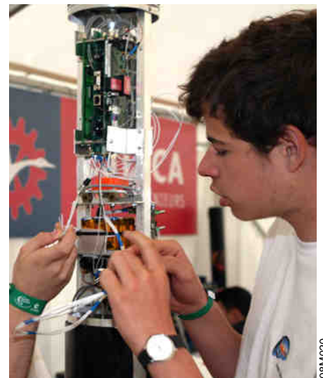
Les jeunes de l'équipe lors de l'intégration de leur module électronique dans l'expérience Perséus FH04.
