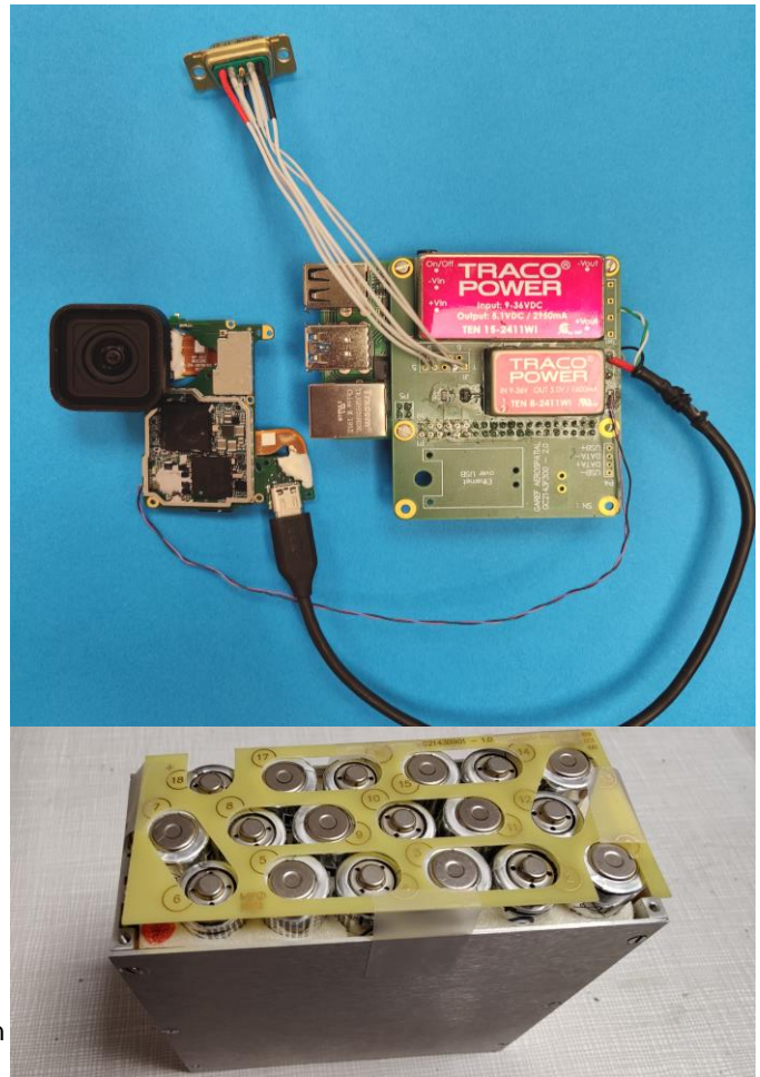
De haut en bas : Système vidéo en cours de test et bloc de piles assemblé avant soudures
