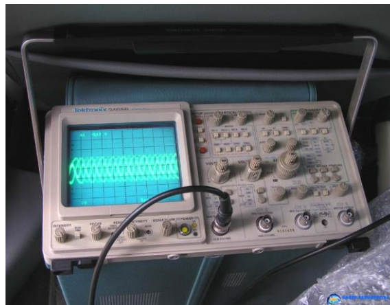
G05O051 Oscilloscope de visualisation du PCM
