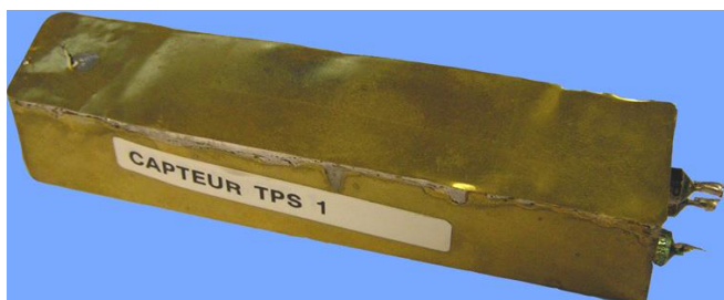
G05Y019 Exemple de boîtier blindé réalisé
