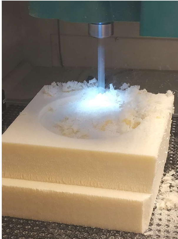
Figure 6 : Usinage d'un couvercle de la nacelle dans un bloc de polystyrène extrudé
