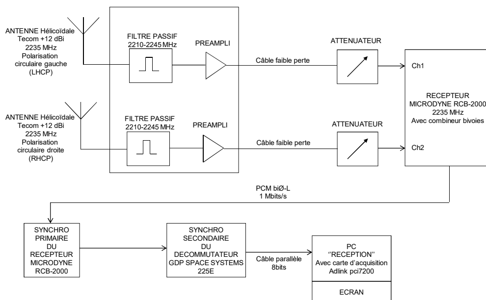
Figure 12 : Synoptique de la station de réception en bande S GAREF (2235MHz,NF<1dB)
