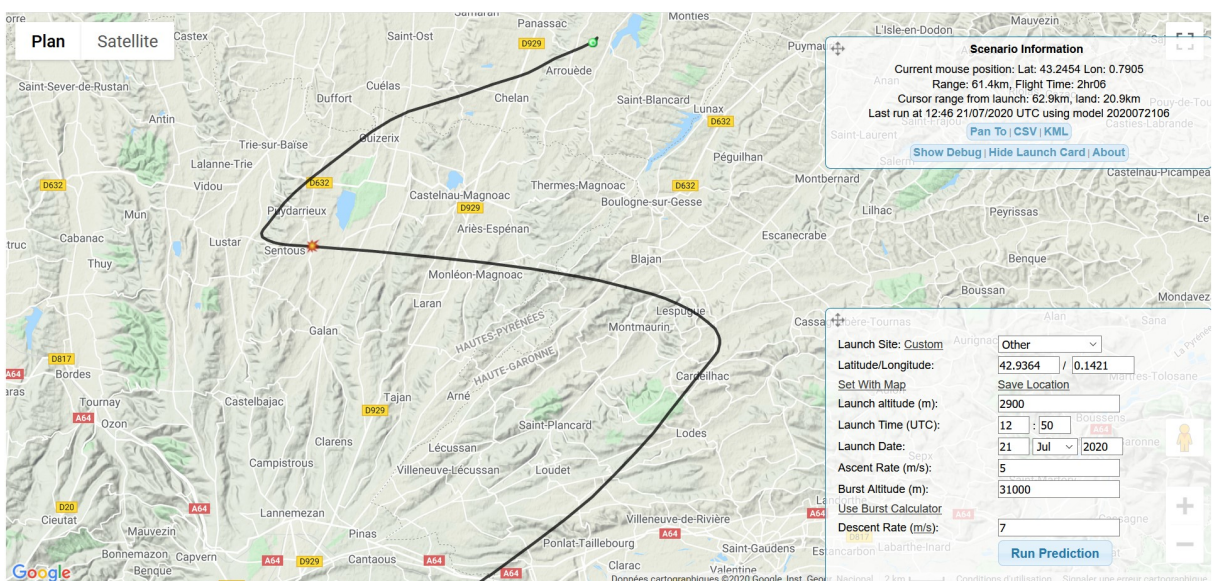
Figure 14 : Une des trajectoires du ballon prévues par le logiciel habhub
